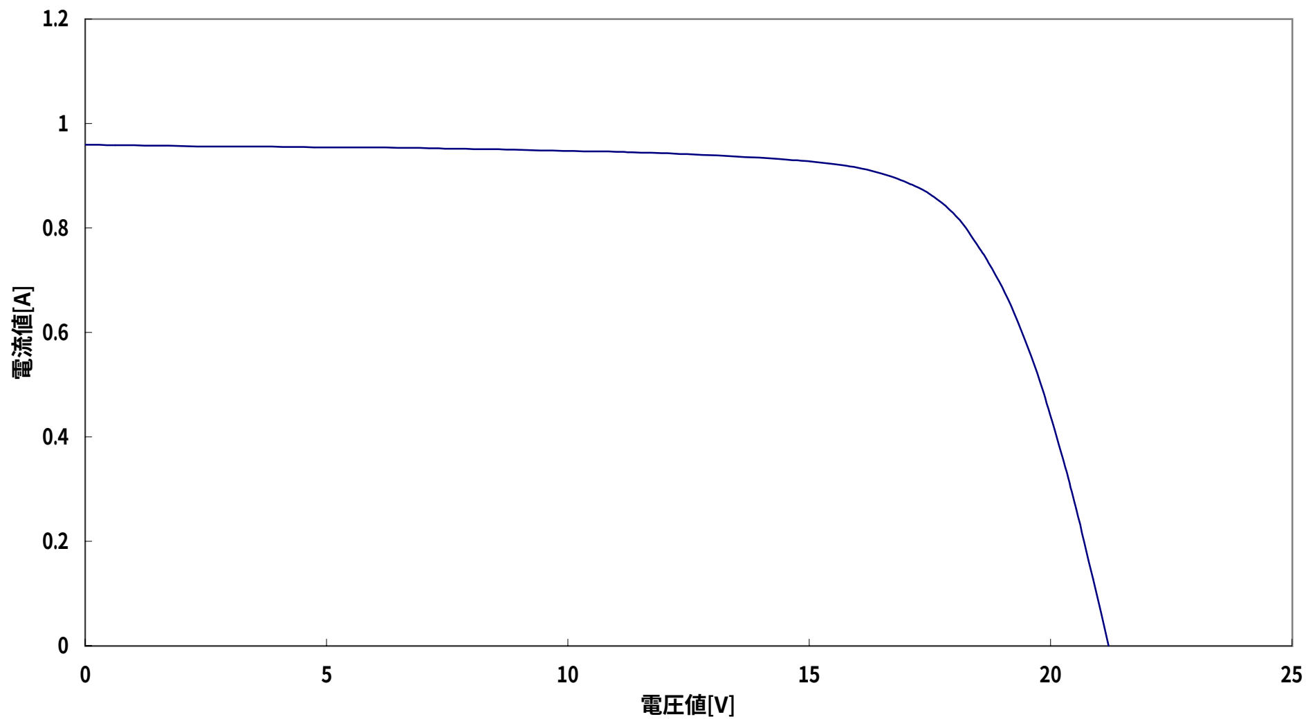
GT434S 出力特性図 @1000W/m 2 AM1.5 25°C
