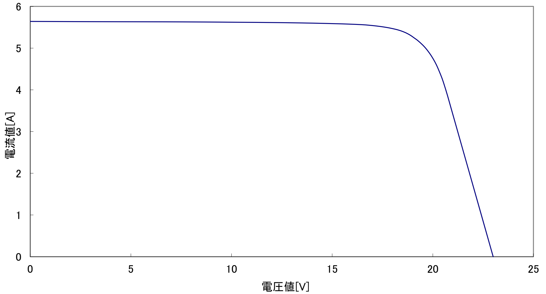
GT-K100 出力特性図 @1000W/m 2 AM1.5 25°C
