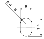
長丸穴詳細
